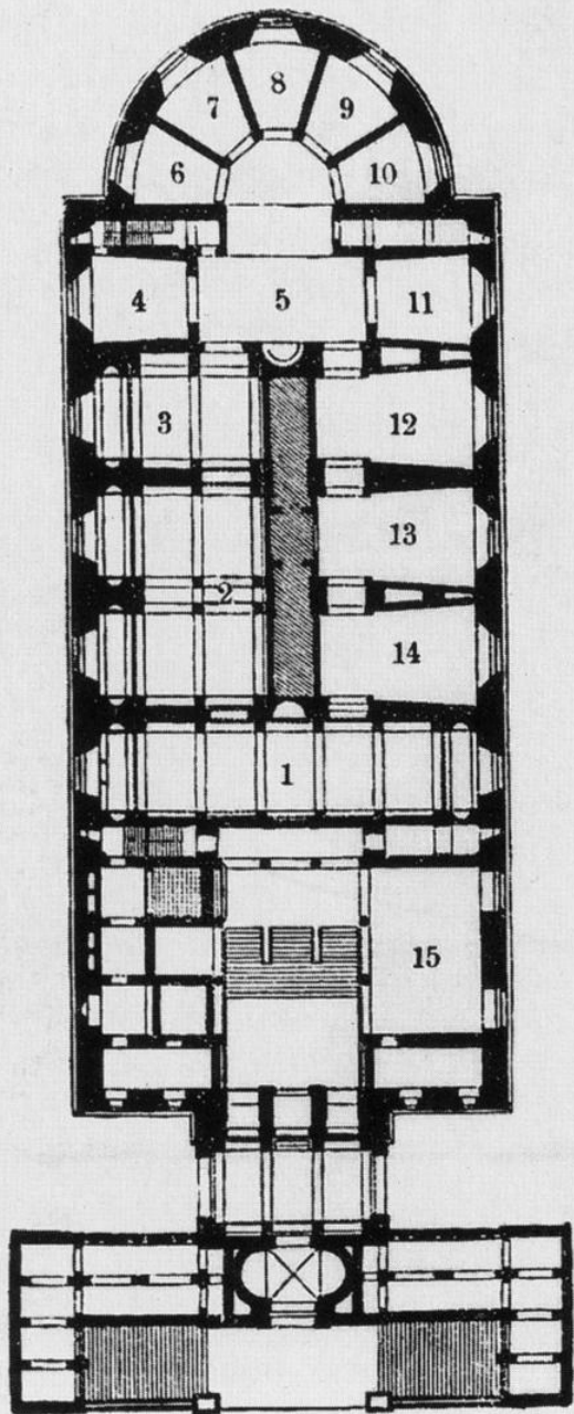
Grundriß des I. Gechoffes.
